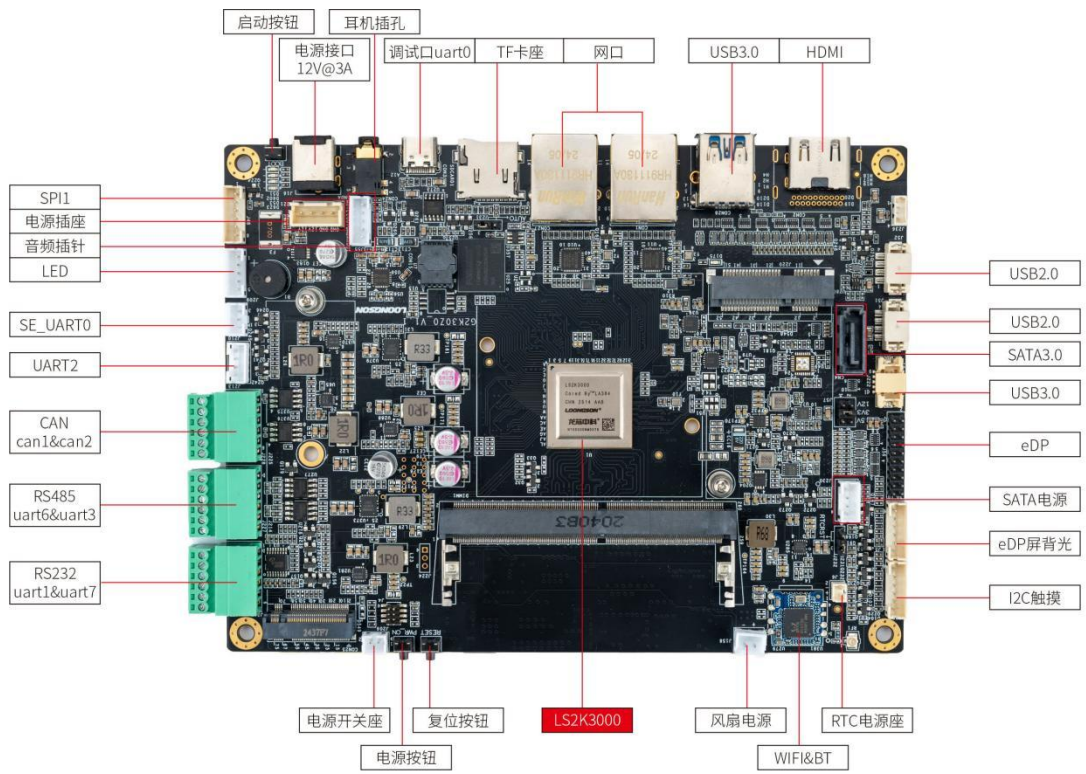
接口图
