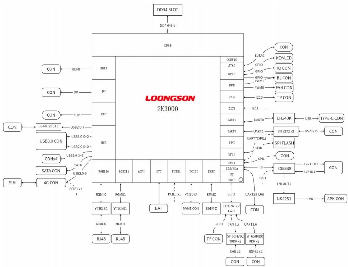
结构框图
